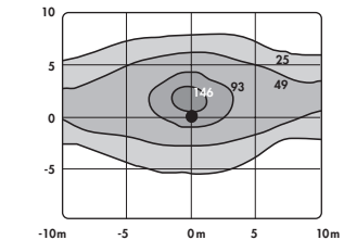
Isolux L.P.H. = 8m
